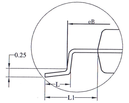
DETAIL: F
